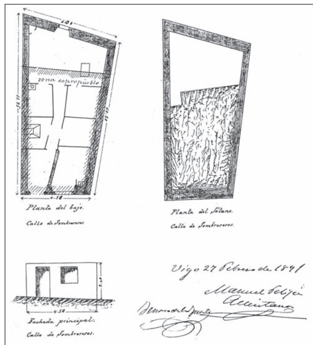
Casa de Ignacio López con frente a rúa Somberreros nº 34. Levantamiento de plano 1891.
