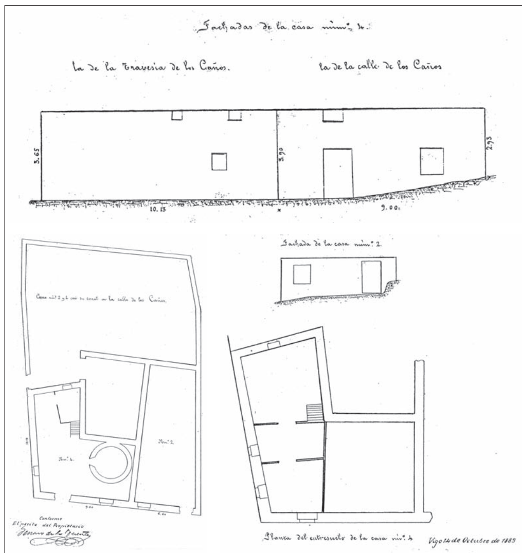
Casa de Constantino Rodríguez Sanmartín con frentes a la rúa de los Caños números 2 y 4 y esquina a la Travesía de los Caños. El doble círculo indica que es un horno de pan. Plano de J. de la F. 1889.
