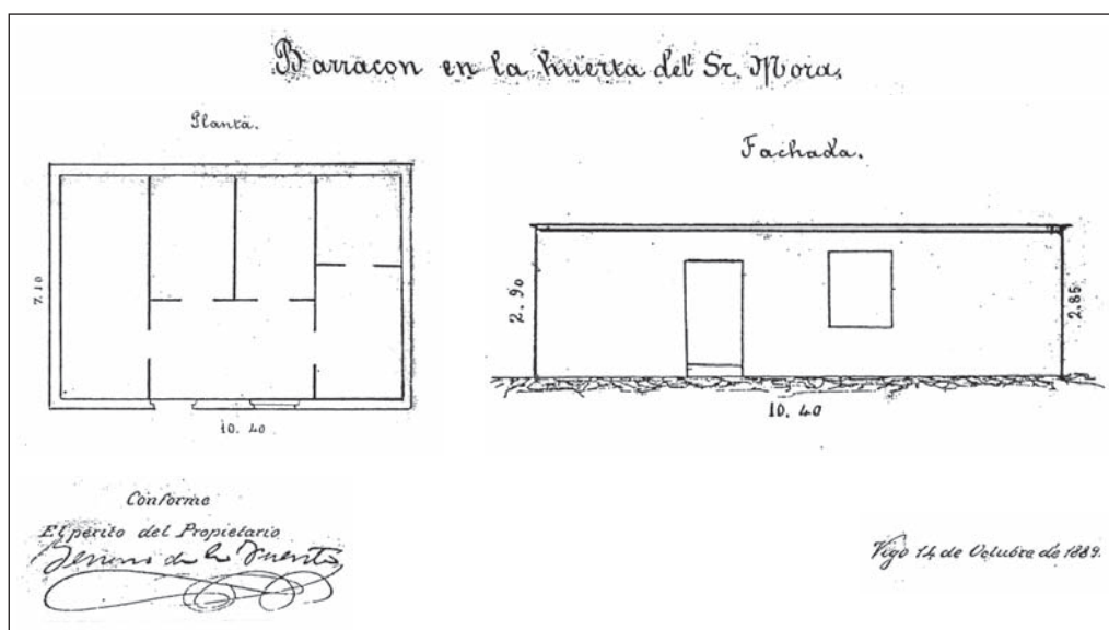
Barracón de Cándida y Augusto, herederos del Sr. Mora, situado en la huerta de la finca. Plano de J. de la F. 1889.
