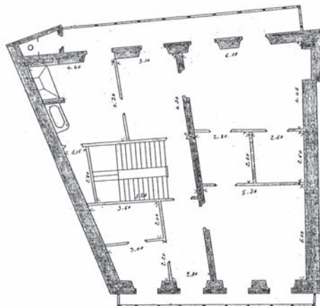
Planta del 2º piso.
