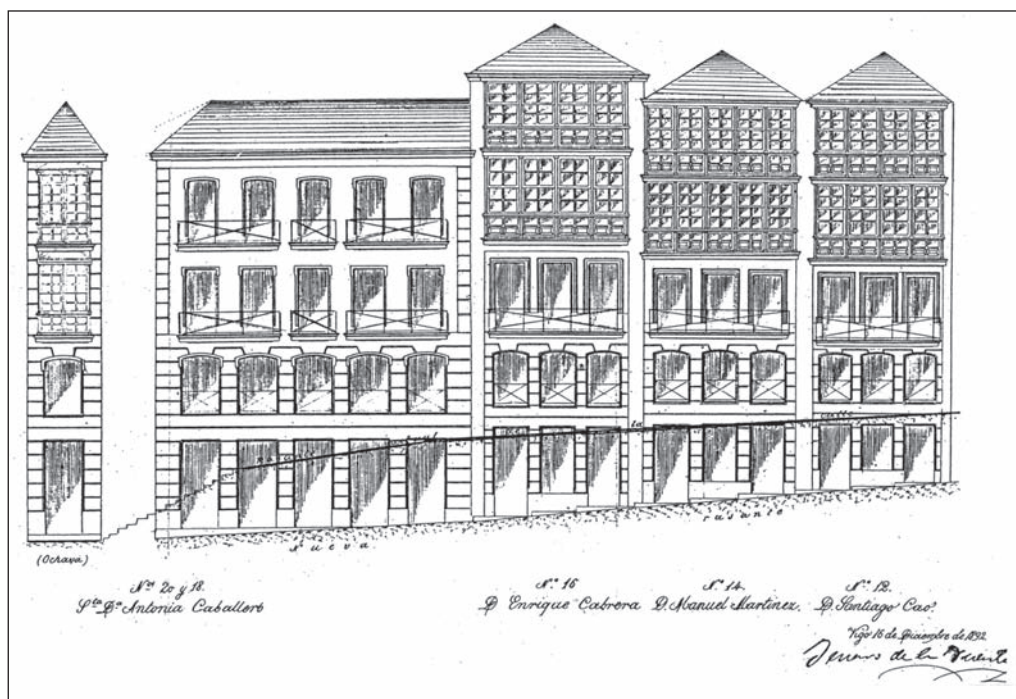
Nueva rasante de la Puerta del Sol eliminando la elevada rúa de la Soledad. Proyecto de Jenaro de la Fuente Domínguez de 1892 con el diseño de las nuevas fachadas (Archivo Municipal de Vigo).
