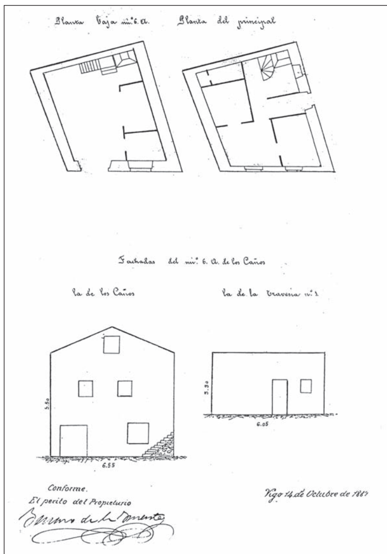
Casa de José Guardado Martínez con frentes a la rúa de los Caños nº 6 A esquina a la Travesía nº 1. Plano de J. de la F. 1889.
