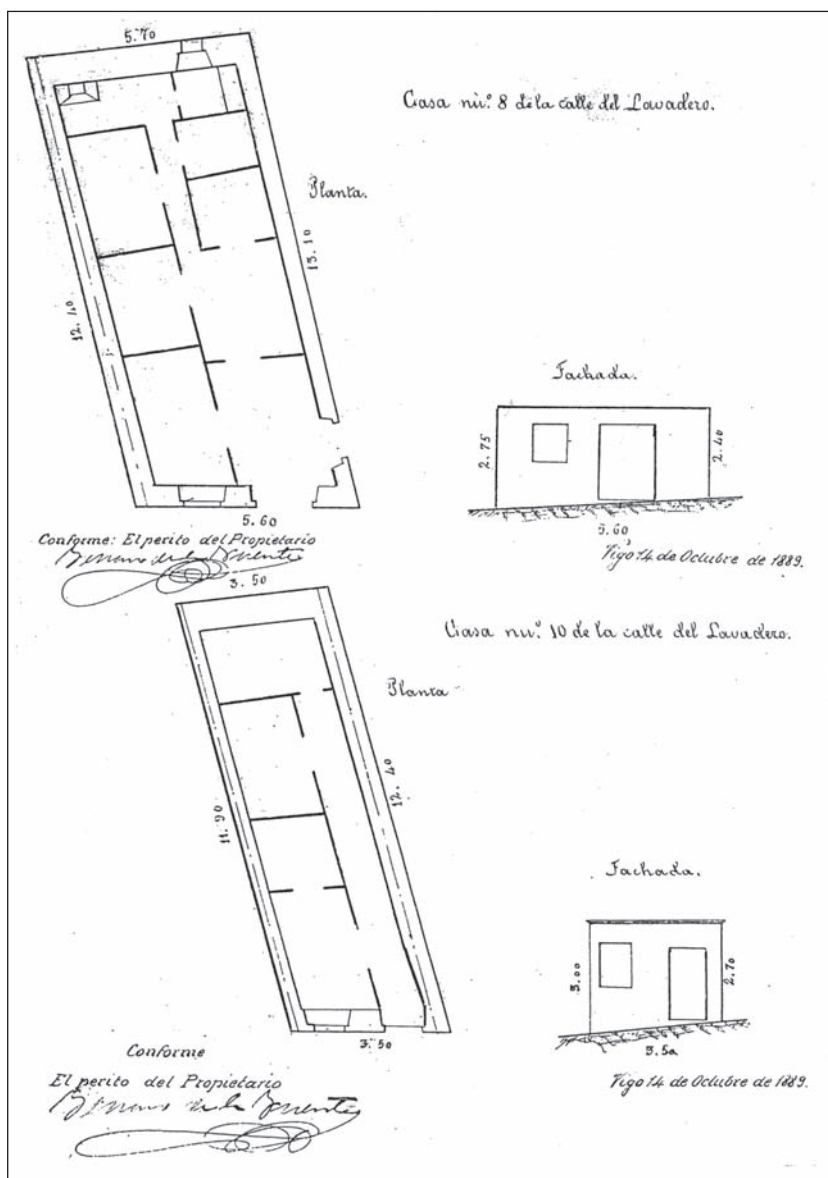
Casas de los herederos de Mora y de Baltasar López Martínez con frente a los números 10 y 8 de la rúa del Lavadero. Plano de J. de la F. 1889.
