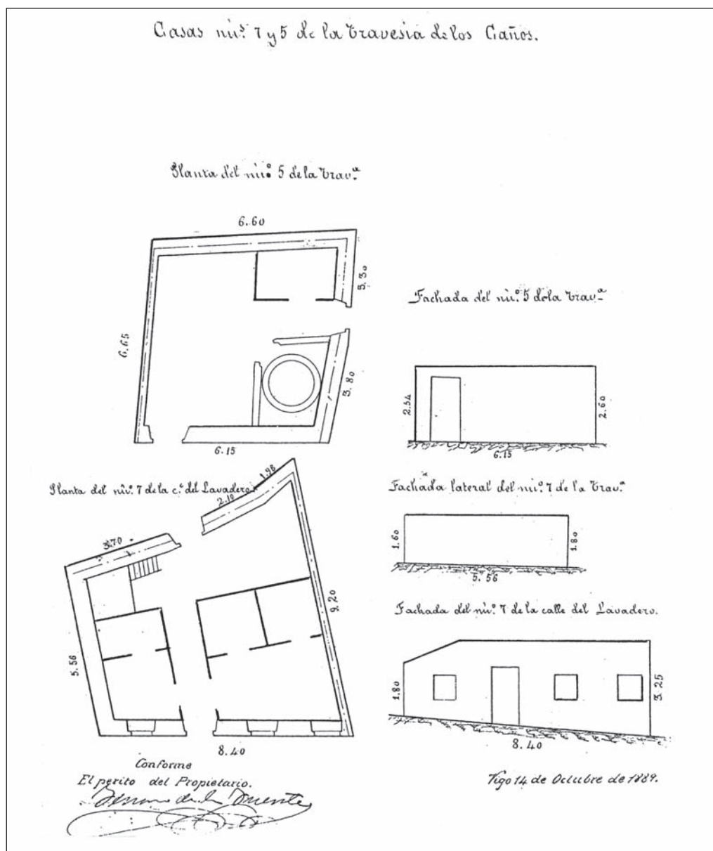
Casas de Ramón Tarrio Reis con frentes a la rúa del Lavadero nº 7 y esquina a la Travesía de los Caños nº 7 y la nº 5 de la citada Travesía. Esta última es un horno de pan. Plano de J. de la F. 1889.
