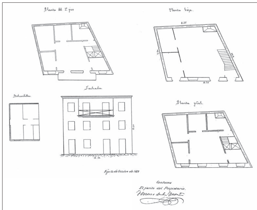
Casa de Gertrudis Fernández y piso de Pilar Baptista con frente a la rúa de los Caños nº 13. Plano de J. de la F. 1889.
