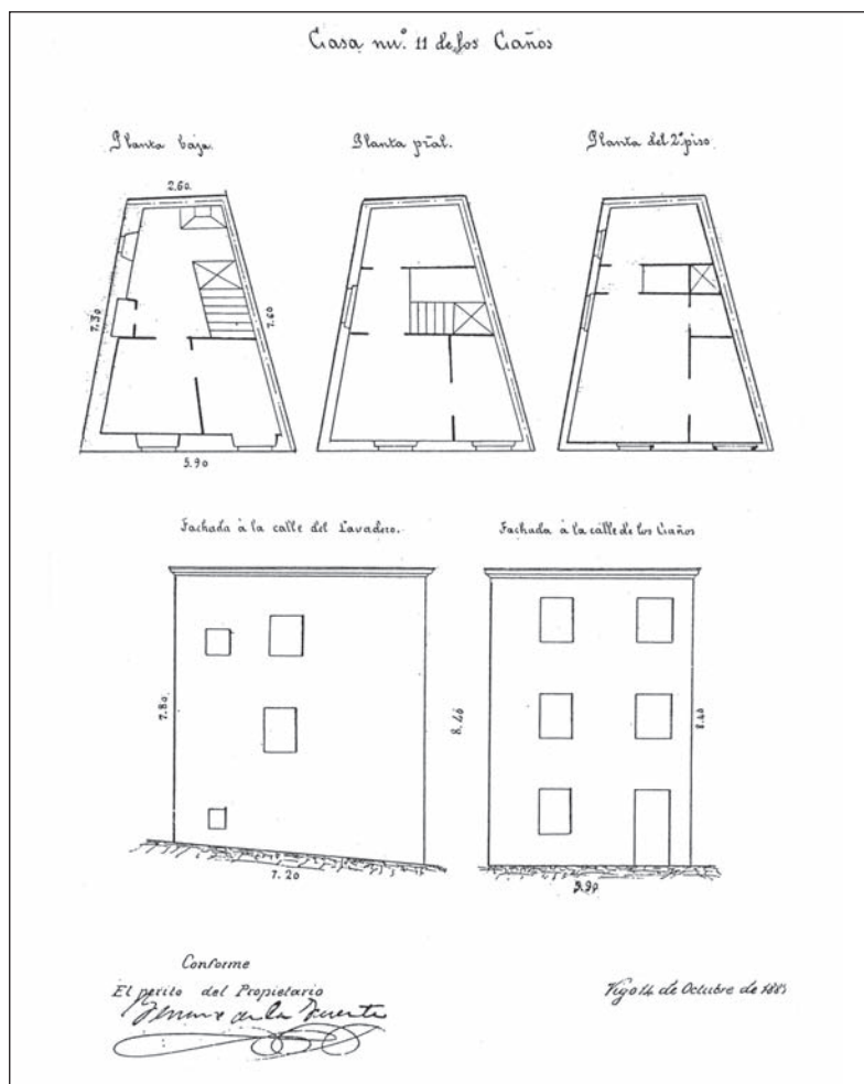
Casa de María Gertrudis Fernández con frentes a la rúa de los Caños n° 11 y esquina a la rúa del Lavadero con el mismo número. Plano de J. de la F. 1889.
