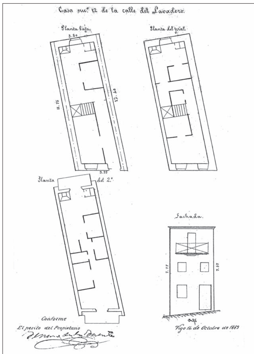
Casa de Ramón Tarrío País con frente a la rúa del Lavadero nº 12. Plano de J. de la F. 1889.
