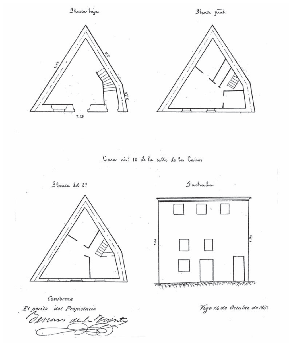
Casa de José González con frente a la rúa de los Caños nº 10. Plano de J. de la F. 1889.
