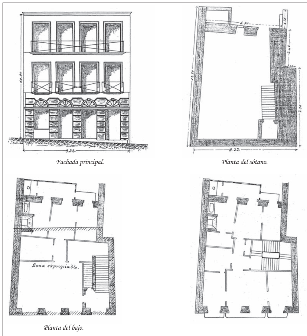
Casa de la viuda e hijos de Núñez con frentes a la rúa Sombrereros nº 32 y con patio en la parte posterior. Levantamiento de plano en 1891.
