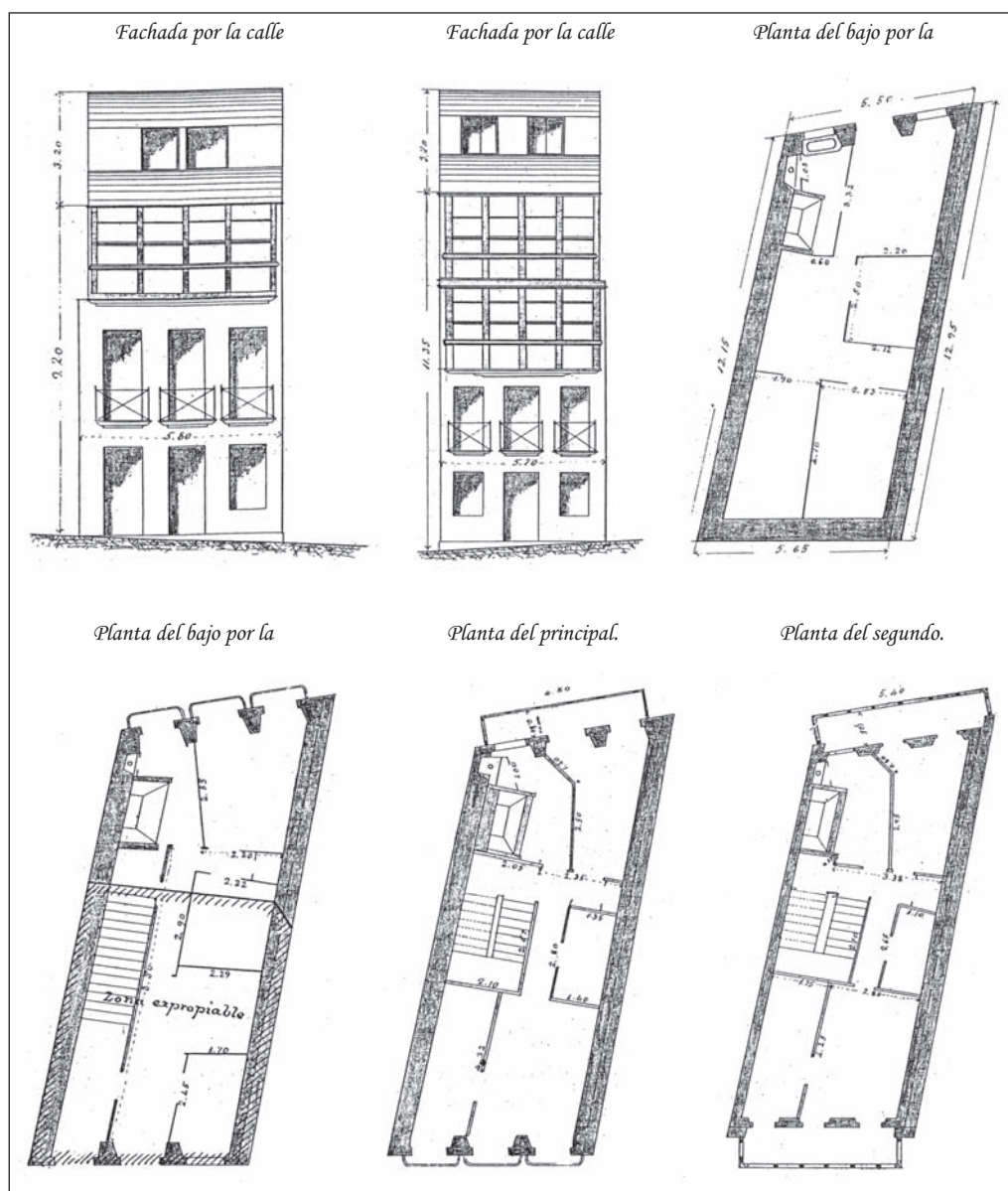
Casa de herederos de Antonio Cordero con frentes a rúa Sombrereros nº 12 y por su lado posterior a la rúa San Vicente nº 7 A.
